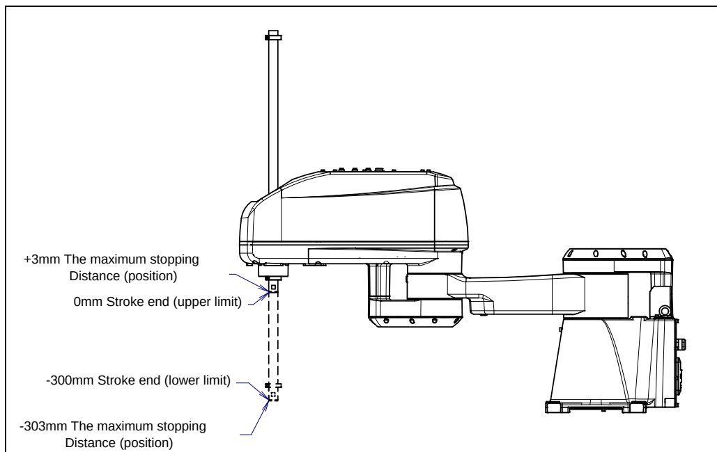
Fig. 3.3 (d) J3-axis motion limit (300mm stroke)
